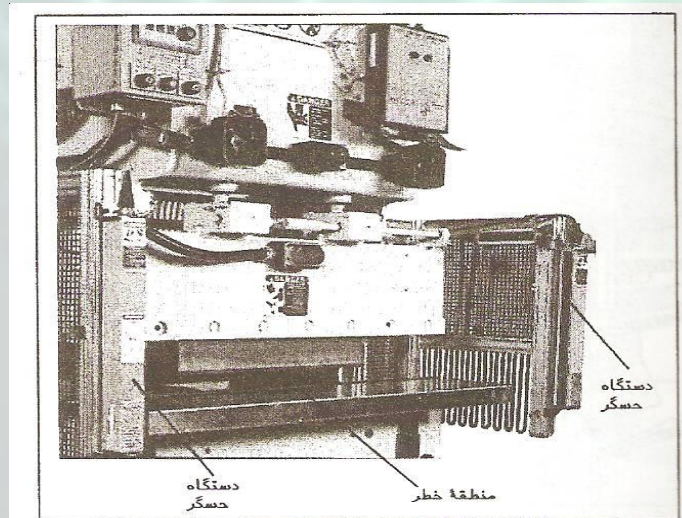
سیستم فتو الکتریک در پرس دارای گارچ با گردش جزئی www.aslandozhealth.blogfa.com tohid alizadeh
