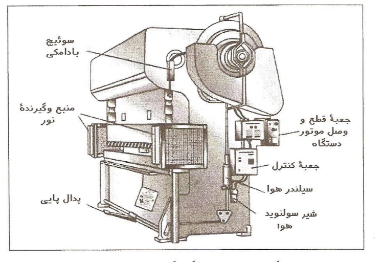
سیستم فتو الکتریک در برک پرس
